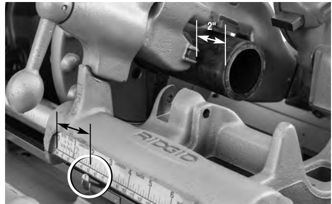
Figura 20 B – Puntero del calibrador de longitud en la longitud deseada
