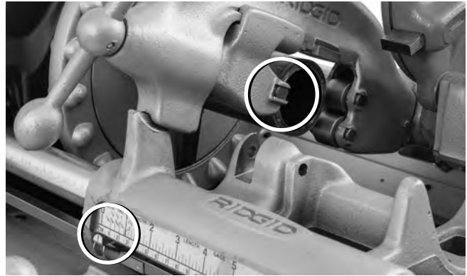
Figura 20 A – Filo de la rueda de corte contra el extremo del tubo. El puntero se coloca en cero (0).
