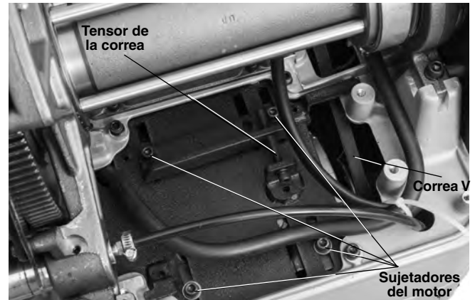
Figura 35 – Tensión de la correa
