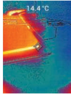
رسم ٥.١. مسح الصورة الحرارية الواضحة (MSX®)
